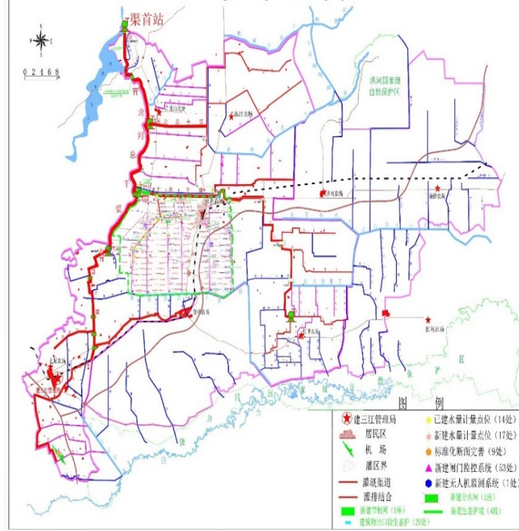
北大荒集团建三江分公司青龙山灌区 深化农业水价综合改革推进现代化灌区建设试点 工程布置图
